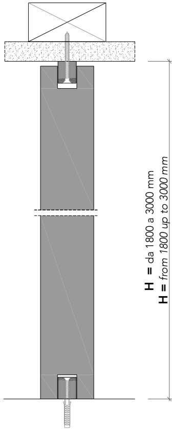
pannello fisso ■ fixed panel
