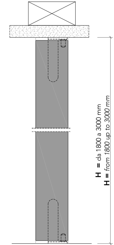
pannello a battente ■ swing panel
